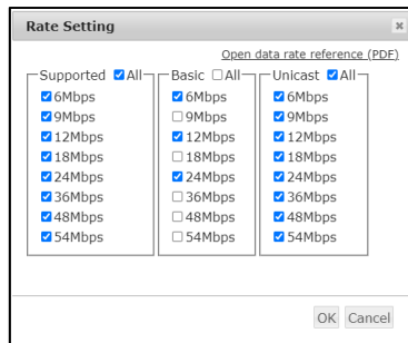
図 7-25 送信レート設定(802.11a/j)
