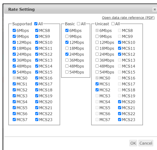
図 7-22 送信レート設定画面(802.11n, ac/5GHz)
