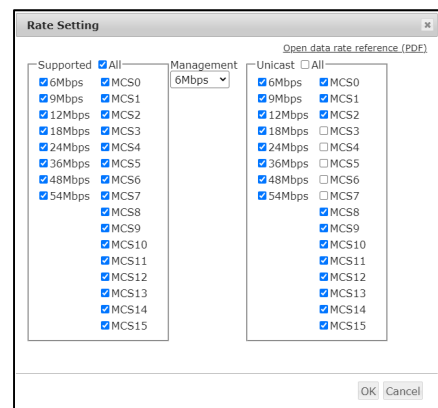
図 7-13 送信レート設定画面(4.9GHz)
