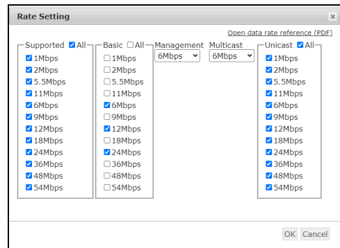
図 7-10 送信レート設定画面(802.11g)
