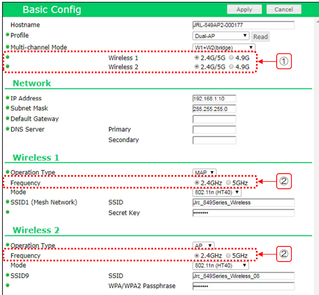
図 4-4 Basic Config 画面関連設定項目
